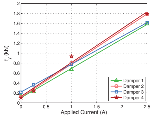
(d) Yield force f_y .
