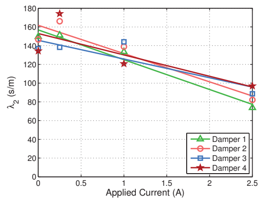
(f) Shaping parameter \lambda_2 .
